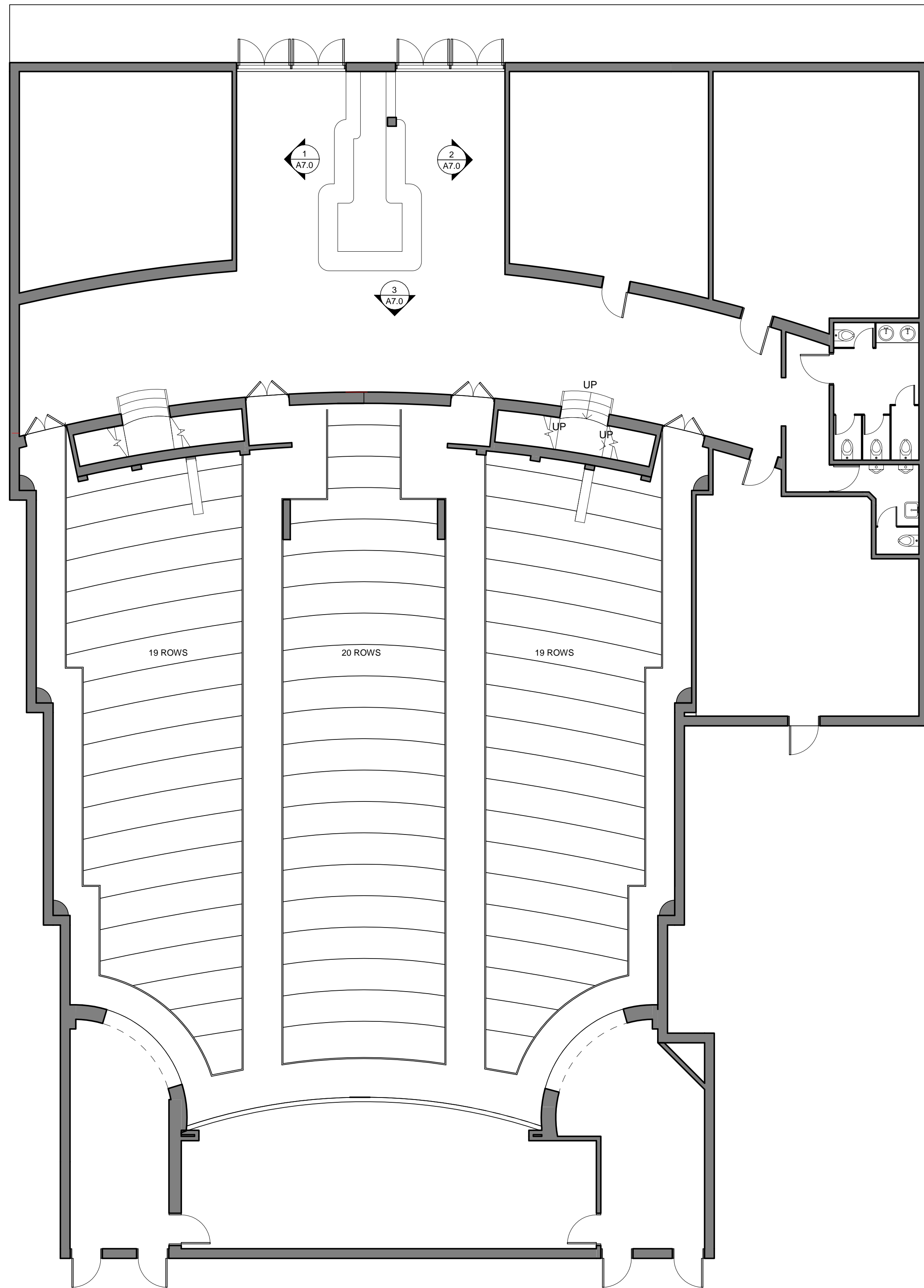
1 MAIN FLOOR DEMOLITION D1.1 SCALE: 1/8" = 1'-0"
