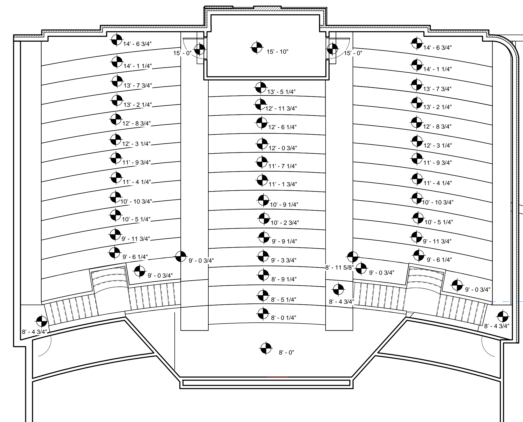
2 SECOND FLOOR DEMOLITION D1.1 SCALE: 1/8" = 1'-0"
