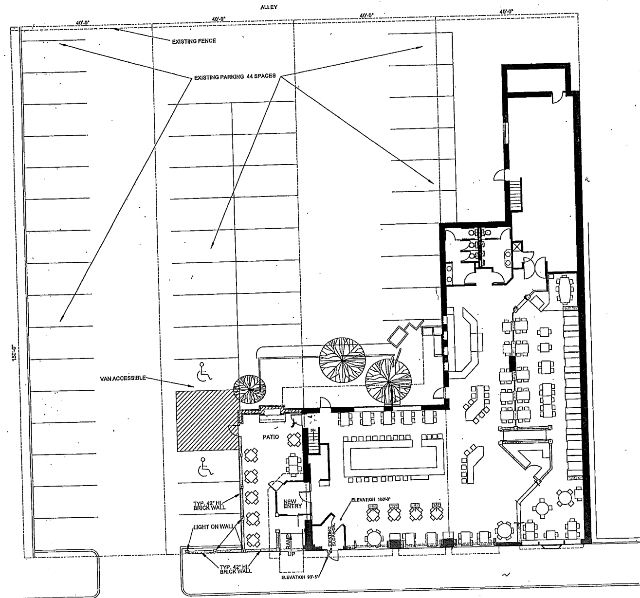
2 SITE PLAN A1.2 SCALE: 1/8" = 1'-0"
